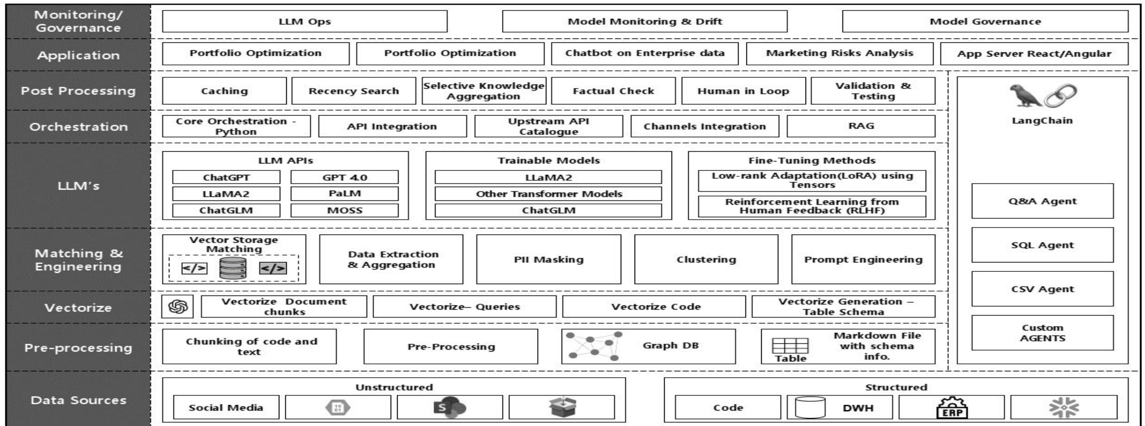
EY Gen AI Framework
