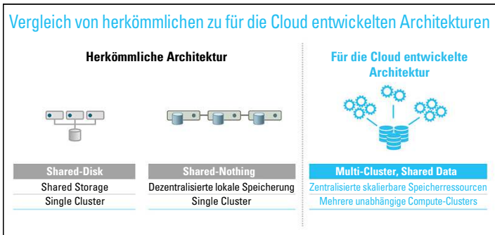
ABILDUNG 5-1: Wie eine cloudoptimierte Architektur die Performance optimiert.
